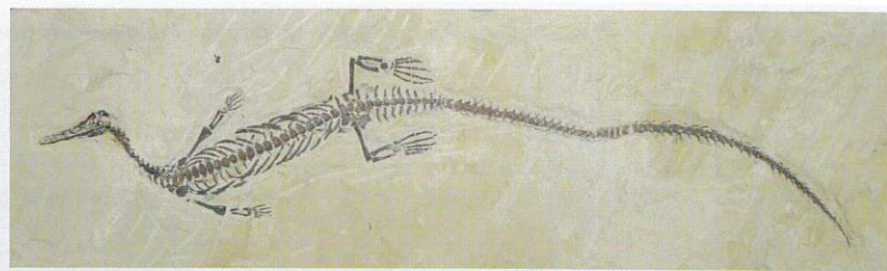
最古の水生は虫類 ブラジル 約 2 億 6 0 0 0 万年前 (一財) 進化生物学研究所
